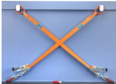
1 Typ XB Nutzlänge pro Zurrstrang = 2,10 m
